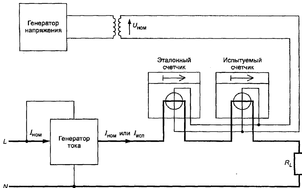
Рисунок А.1 — Схема испытательной цепи (справочная)
